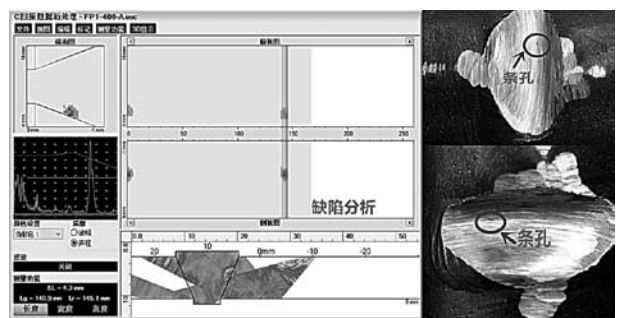
图 9 FP1-406 焊口缺陷分析过程示意图 及打磨缺陷图
